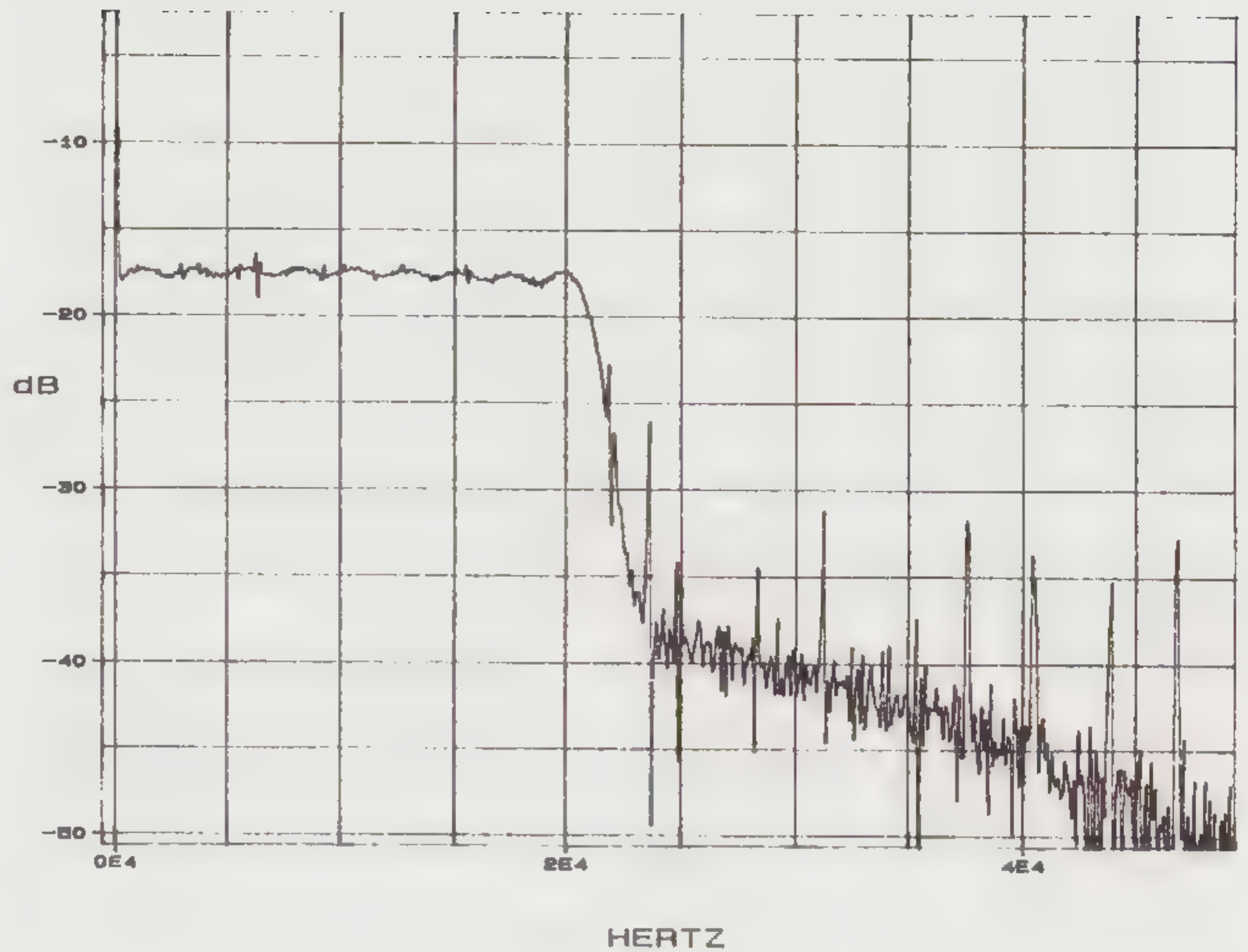
Figuur 2. De Akai gemeten tot 50 kHz
